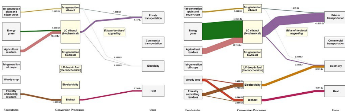
Figure reprenant la production globale de biomasse, ses conversions et ses débouchés énergétiques pour la référence « business as usual » (à gauche) et avec un prix du carbone (hors application au changement d'usage des terres, à droite)
