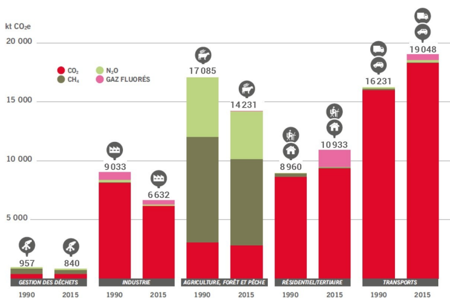
Évolution des émissions de gaz à effet de serre par secteur et par gaz, entre 1990 et 2015
