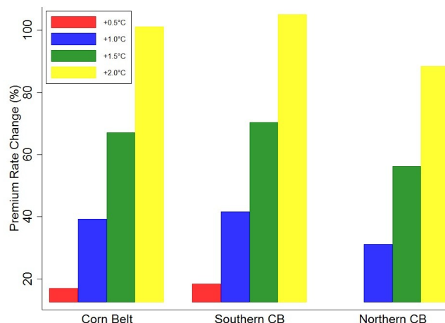
Estimations de l'évolution des primes d'assurance selon quatre scénarios climatiques (assurance du maïs, 90 % de couverture, évolution en %, pour a) la zone de production principale - Corn Belt , b) le Sud et c) le Nord de cette zone)
